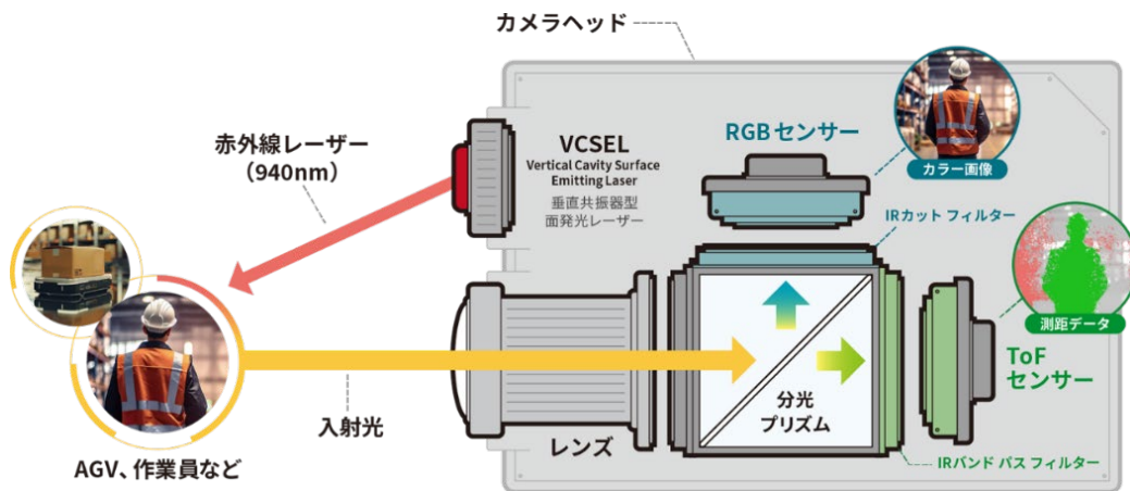
<当社センサーフュージョンカメラ概念図>
